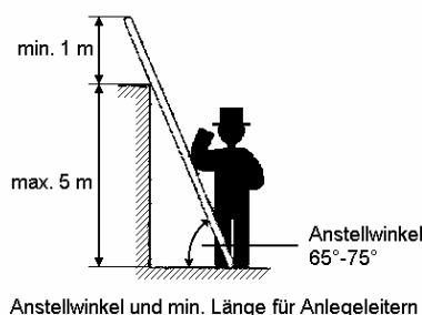
Anstellwinkel und min. Länge für Anlegeleitern
